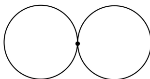
FIGURA 12. Un wedge di due circonferenze
