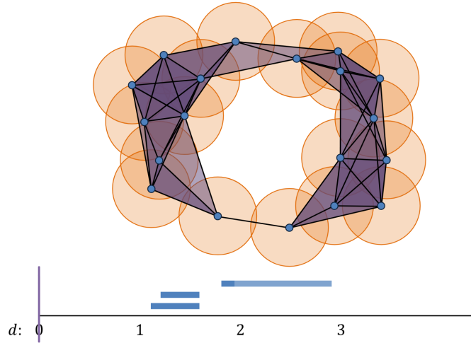
FIGURA 9. Codice a barre formatosi all'aumentare di d
