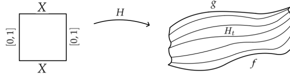
FIGURA 4. Omotopia come interpolazione tra una mappa f a una mappa g
