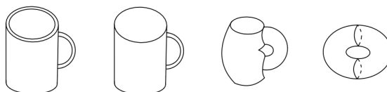
FIGURA 3. Un omeomorfismo tra una tazza ed un toro
