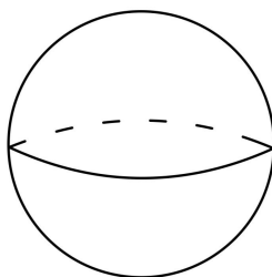
FIGURA 11. La sfera S^2
