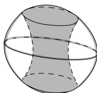
FIGURA 14. Un retratto per deformazione di Y
