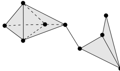
FIGURA 6. Complesso simpliciale
