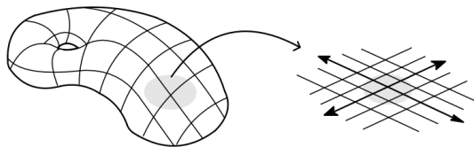
FIGURA 2. Una varietà 2-dimensionale
