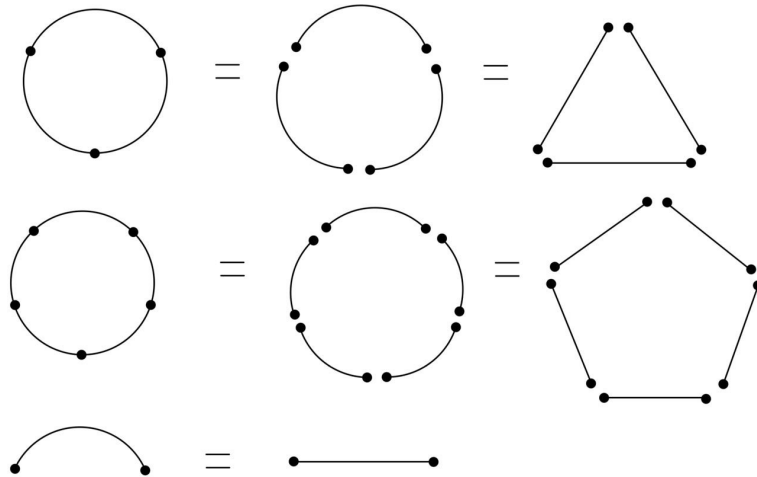
FIGURA 7. Possibili triangolazioni della circonferenza S^1
