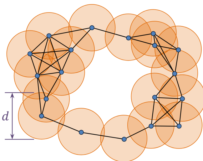
FIGURA 8. Algoritmo esposto per una generica nuvola di punti
